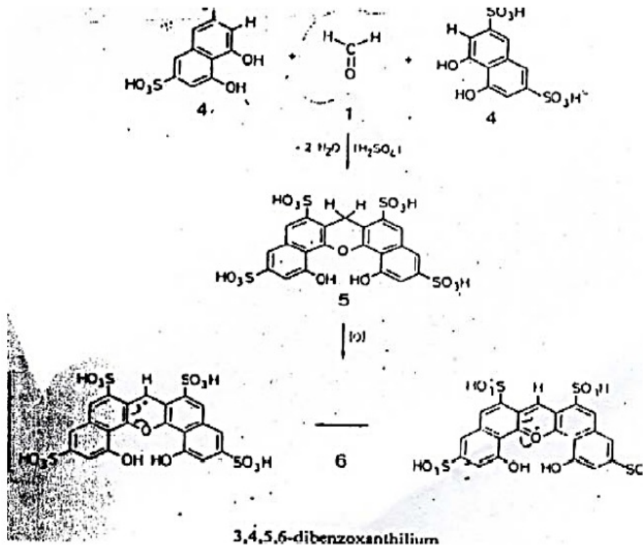
Gambar 5. Reaksi Asam Kromotropat dengan Formaldehid
