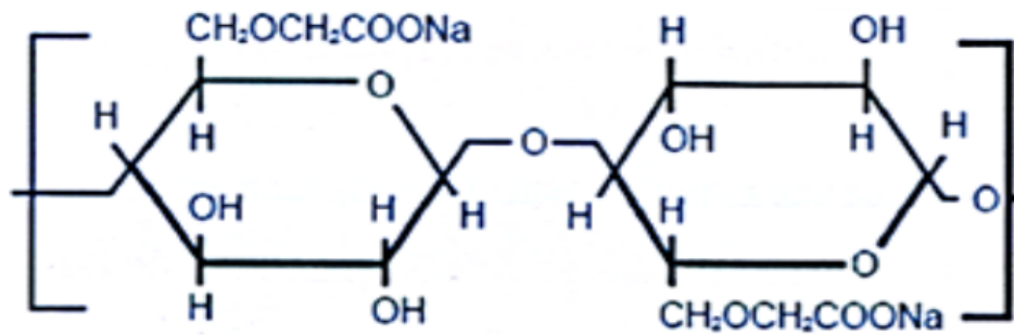
Gambar 2. Struktur CMC
